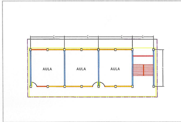
F2: Planta Arq. Edificio B
