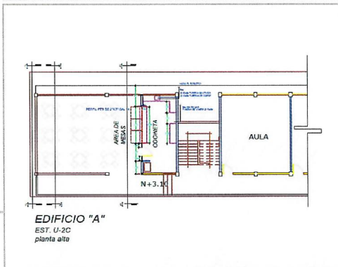
F3: Planta Arq. Nevería
